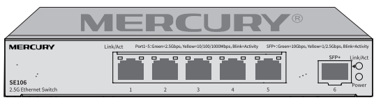
图2-2 SE106前面板示意图
