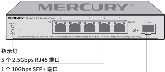
图 2-4 SE106P 前面板示意图
